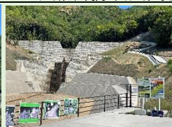
国直轄の砂防堰堤整備
